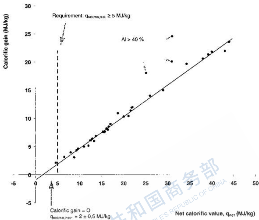
图 B. 2—热量增量和 Q_{net} 的函数关系适用于表 B. 1 的包装成分或组份
