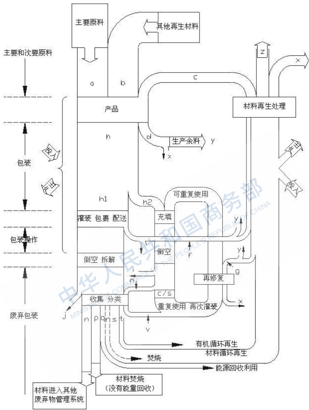
图 1 包装和包装材料流程
